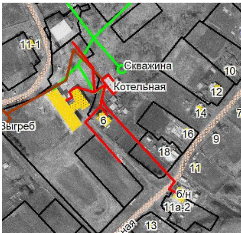
Рисунок 5 – Существующая зона действия котельной № 2 д. Мозжуха
